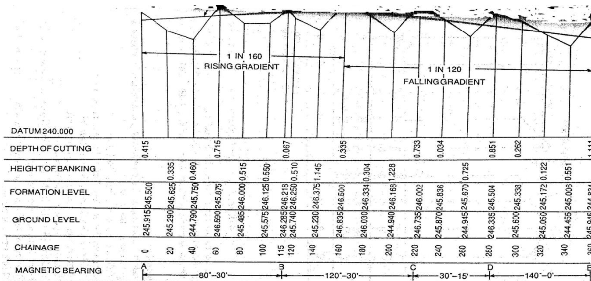
LONGITUDINAL SECTION Fig.
